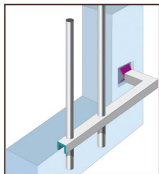
F/1 scellement en façade
