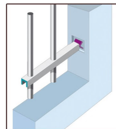
T/1 scellement en tableau
