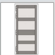
4 paumelles soudées 5 omégas raidisseurs
