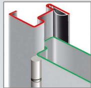
Anti-dégondage par tenon-mortaise avec joint
