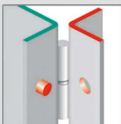
3 renforts de paumelles soudés
