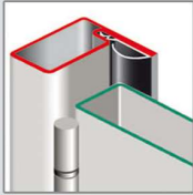
Huisserie tubulaire avec joint
