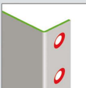
Perçage/ fraisage du blindage
