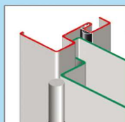
Huisserie rénovation tenon-mortaise BDF
